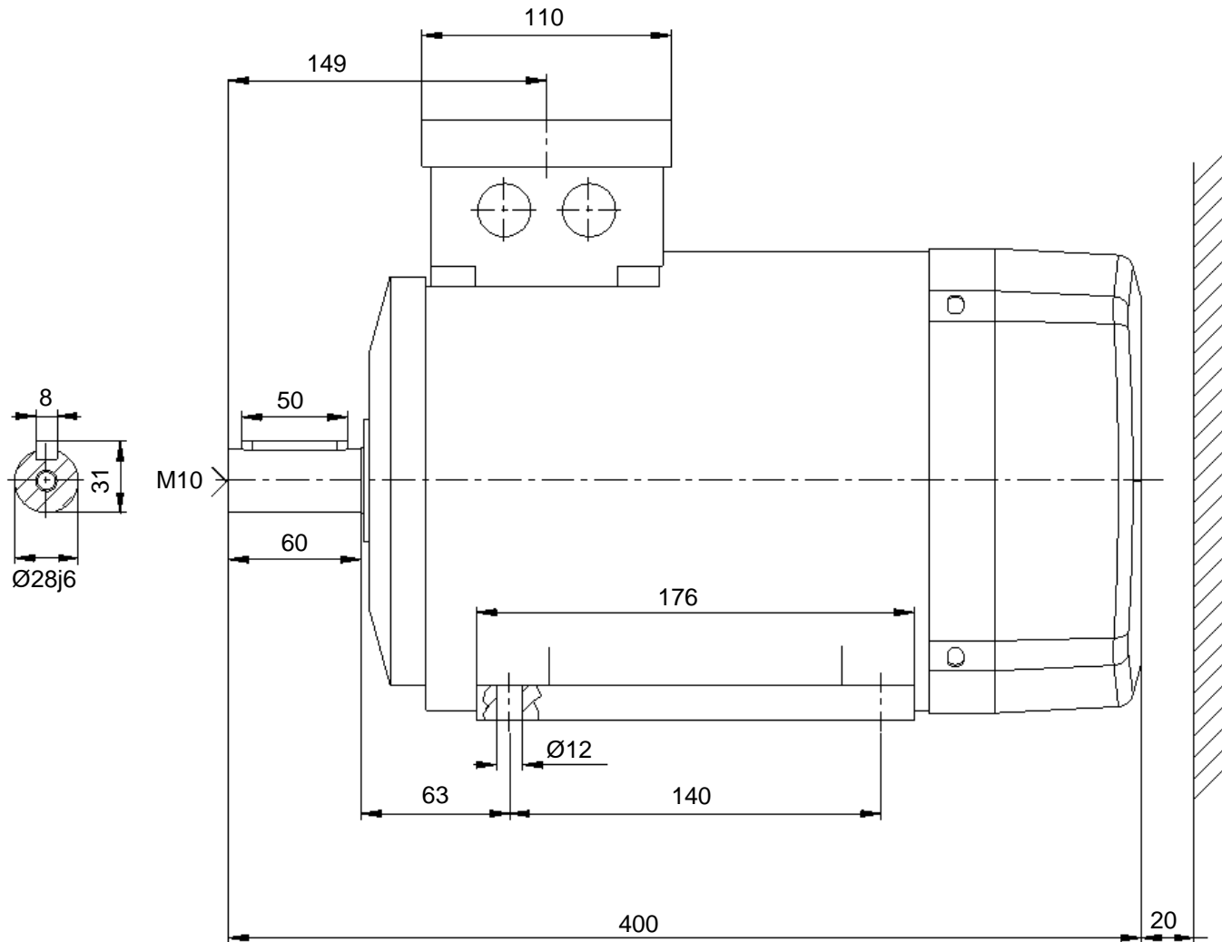
Maßblatt - #303422 - KTE3 100 L 4 KT FL IE3 in Angebot An155696 Position 1 Kabelverschraubung: 2x M25x1,5
