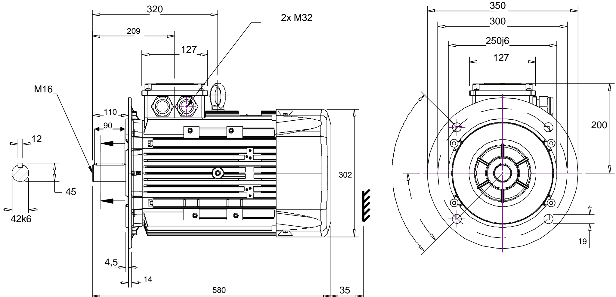
Maßblatt - #300737 - KTE2W 160 M x 2 KT FL IE3 in Angebot An152310 Position 1
